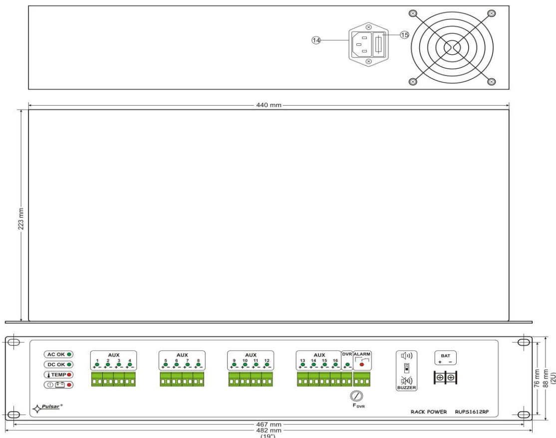
Rys.3. Widok zasilacza.
